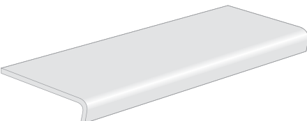
elemento scala piegato TME44SCALA 60 60x32,5xh5
